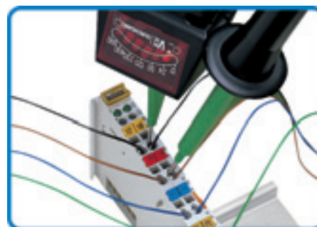
Проверка прохождения сигнала при подсоединенных проводниках
