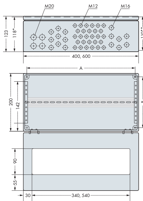
Размеры в мм * внутренние размеры ** от верхнего края рельса DIN 35
