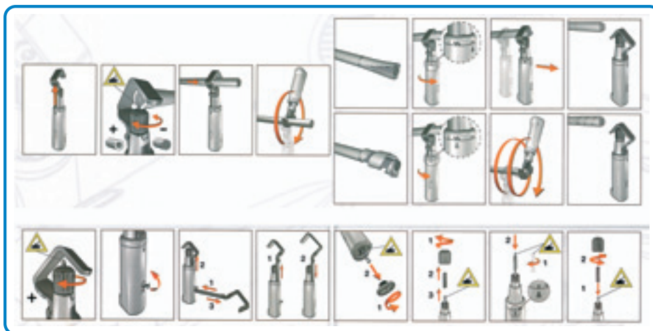
Инструкция по эксплуатации инструмента для зачистки кабелей 206-174
