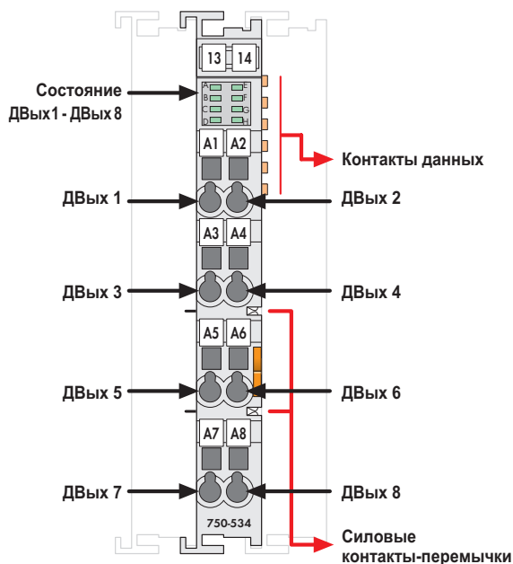
Рис. для серии 750/Технические данные см. на стр. 24/Поставляется без мини-акторных маркеров WSB Маркировку для серий 750/753 см. на стр. 12 - 13/14 - 15
