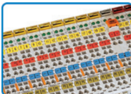
Маркировка зажимных элементов цветными миниатюрными маркерами WSB
