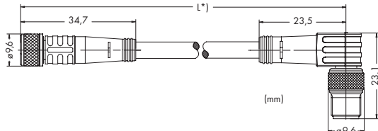
Гнездо M8
