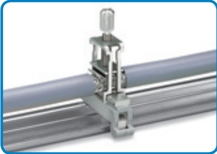
Держатель с заземляющей ножкой 45 мм/1,772 дюйма в длину, шинопровод под углом 90° к рельсу Код 790-113
