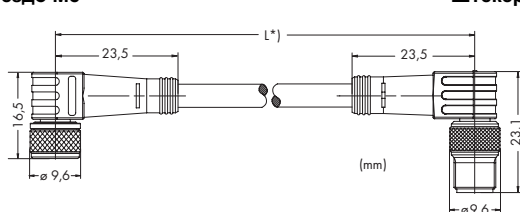
Гнездо M8
