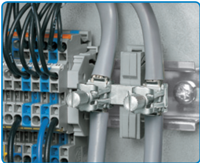
- Держатель с заземляющей ножкой, шинопровод параллельно рельсу
