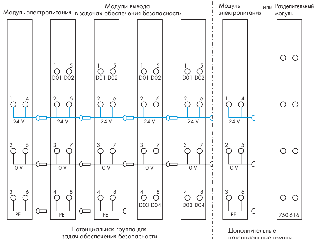
Модуль безопасного переключения/ модуль безопасности
