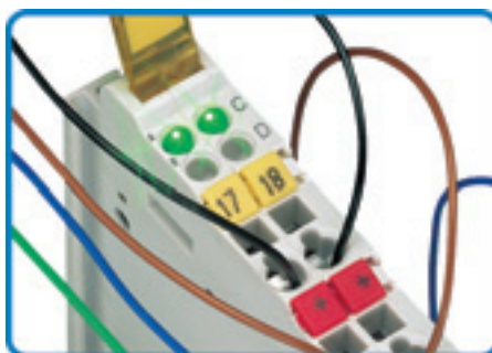
Диагностика и индикация статуса с помощью светодиодного индикатора для надежного запуска и контроля системы
