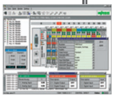
Пример конфигурирования с помощью WAGO-I/O-CHECK
