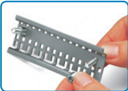
Использование распорной втулки со специальным перфорированным монтажным рельсом
