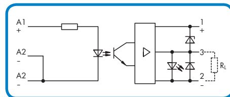
3-проводное выходное PNP-переключение
