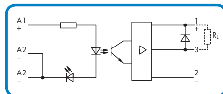
3-проводное выходное NPN-переключение
