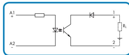
2-проводной выход
