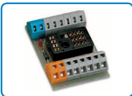
Релейный цоколь
