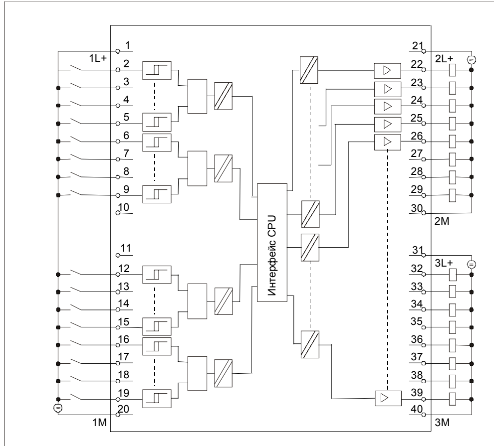
Рис. 7-4. Принципиальная схема встроенной цифровой периферии CPU 313C/313C-2/314C-2
