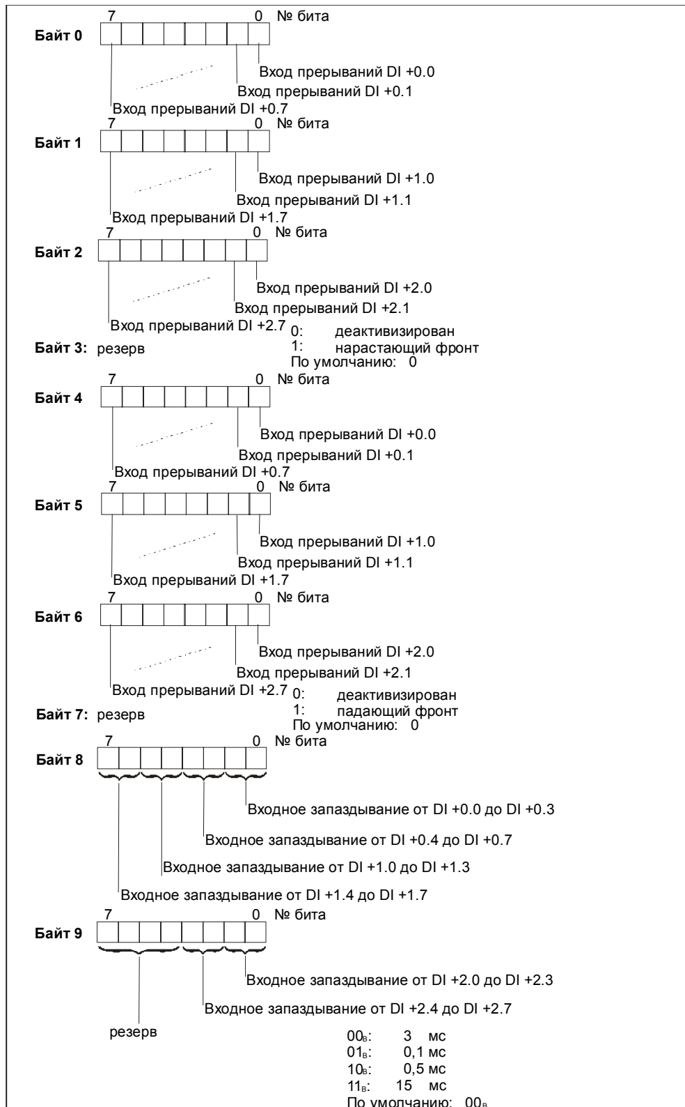
Рис. 7-13. Структура набора данных 1 для стандартного цифрового входа и входов прерываний (длина 10 байт)
