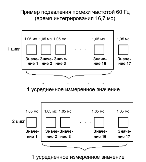
Рис. 7-12. Подавление помехи частотой 60 Гц
