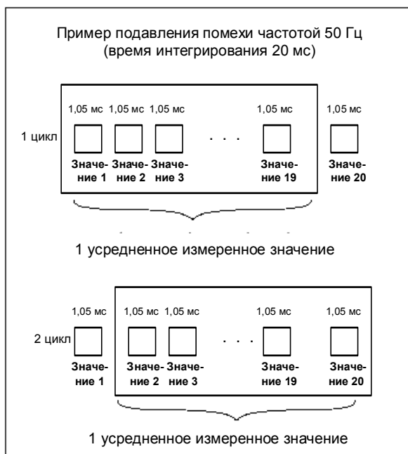
Рис. 7-11. Подавление помехи частотой 50 Гц
