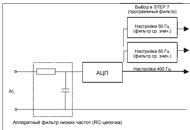
Рис. 7-10. Принцип подавления помех с помощью STEP 7
