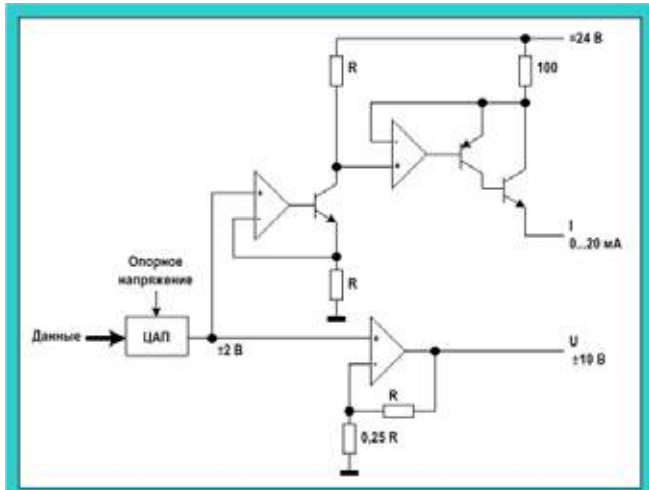
Выходные каскады модулей 6ES7 232-0HB22-0XA0 6ES7 232-0HD22-0XA0 6ES7 235-0KD22-0XA0
