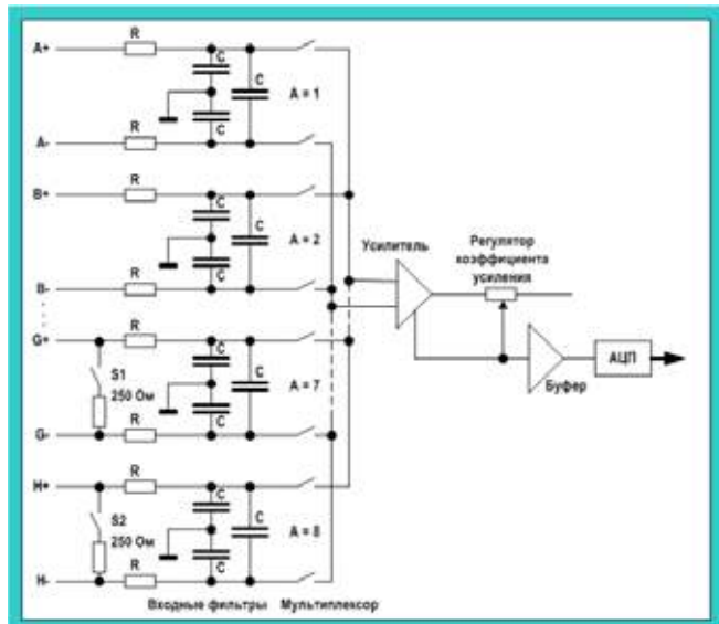
Входные каскады модуля 6ES7 231-0HF22-0XA0
