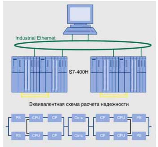
Обмен данными через кольцевую сеть Industrial Ethernet с использованием стандартных схем включения коммуникационных процессоров
