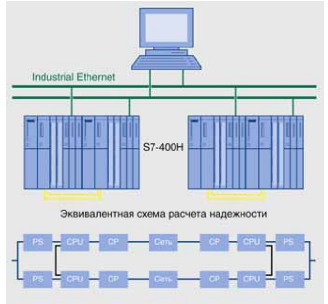
Обмен данными через резервированную сеть Industrial Ethernet с использованием стандартных схем включения коммуникационных процессоров
